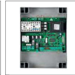
Uitgebreide motorsturing 230-400V met display voor 1 schuifpoortmotor. Met ingebouwde ontvanger 433,92 Mhz.
