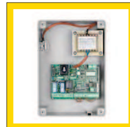
Eenvoudige motorsturing 24 Vdc Ingebouwde ontvanger 433,92 Mhz Programmering van diverse logische functies via display
